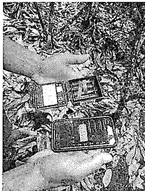
Fotografía 3. Vincular el audiomoths a la aplicación del celular para su encendido.
